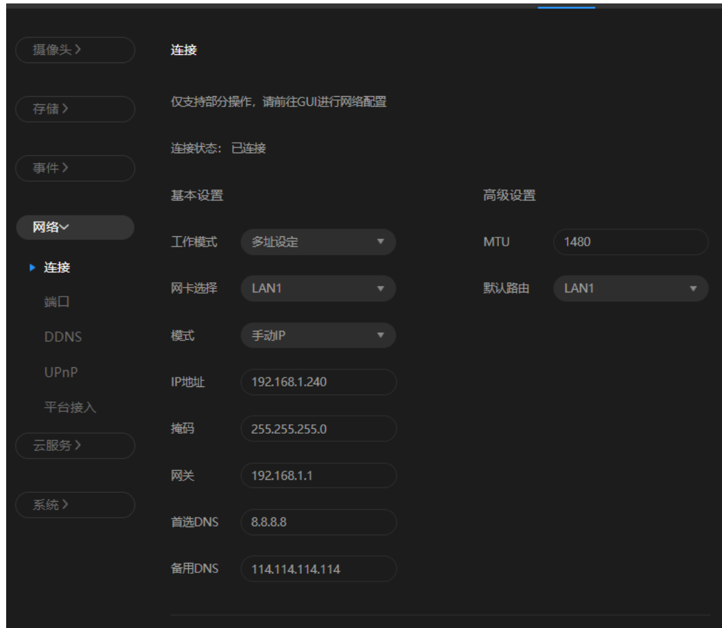
图 5-21 设置 - 网络 - 连接 - 多址设定
